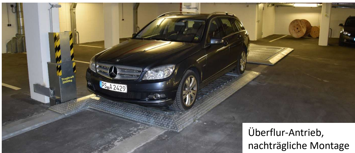
Überflur-Antrieb
