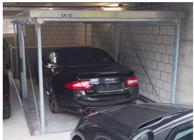
Versenkgarage mit versenktem Ständer. Oberer Belag: Betonierete Wanne
