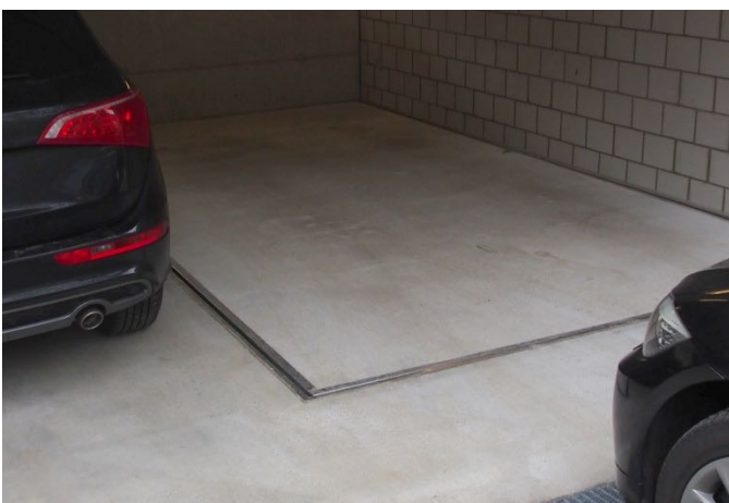
Versenkgarage mit versenktem Ständer. Oberer Belag: Betonierete Wanne
